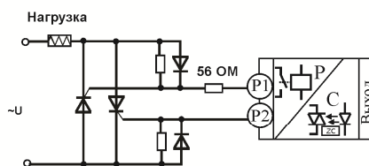
Подключение внешних тиристов
