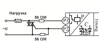
Подключение внешнего симистора
