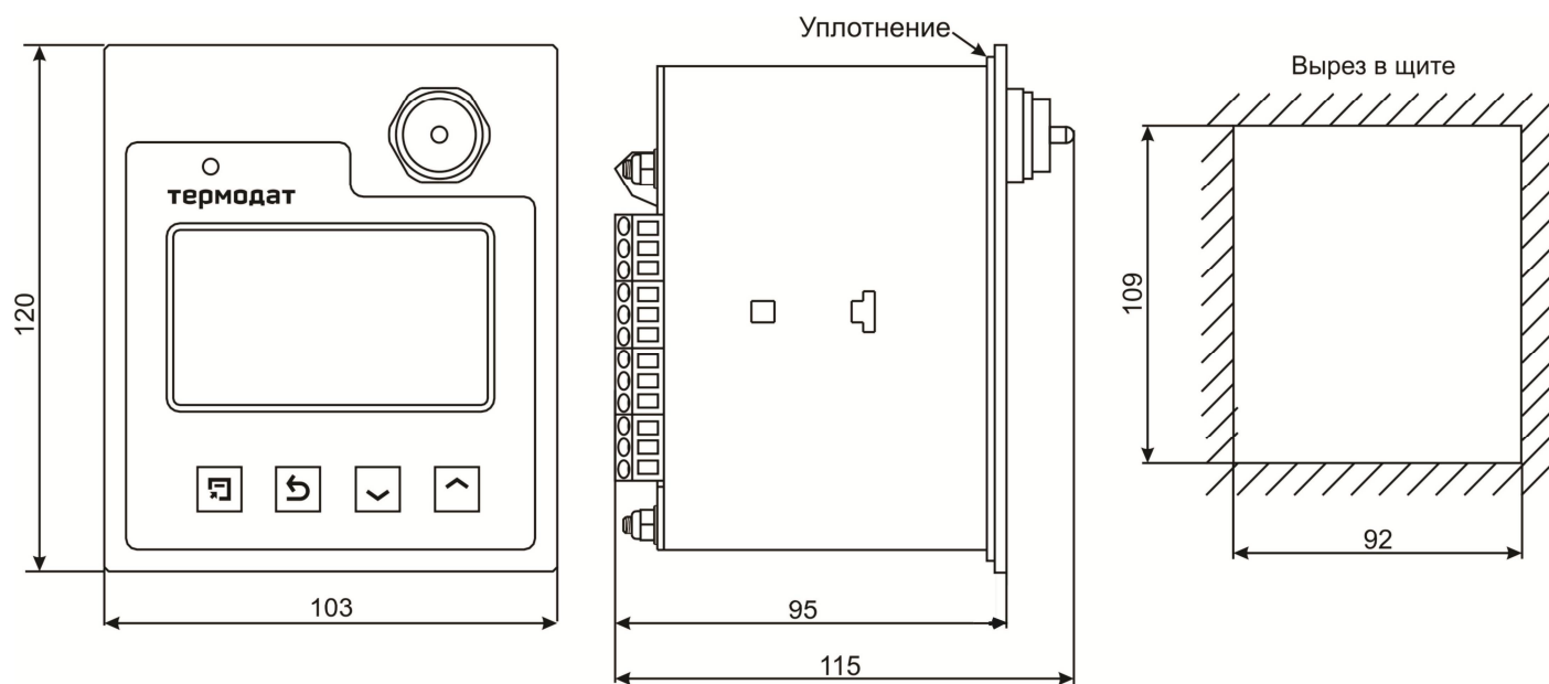
Рисунок 14 – Габаритные размеры прибора Термодат-16E6/...../IP67пп или Термодат-16E6-A7
