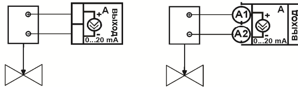
Подключение задвижки с электроприводом
