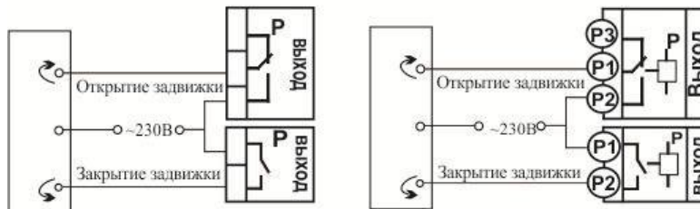
Подключение электрозадвижки
