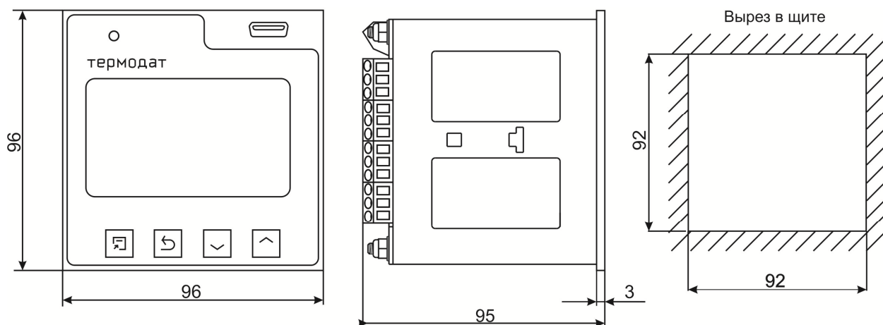
Рисунок 13 – Габаритные размеры прибора Термодат-16E6/...../(F) или Термодат-16E6-A-(F)-(Eth)
